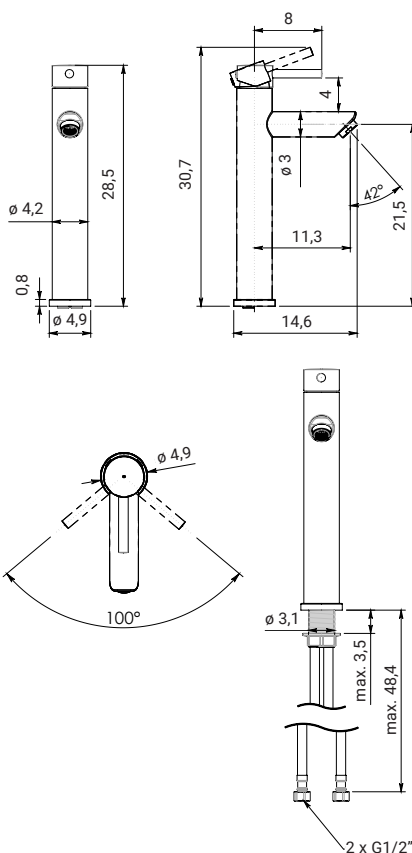
Miscelatore lavabo alto High basin mixer
