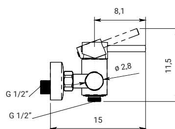
Miscelatore esterno doccia Wall-mounted shower mixer
