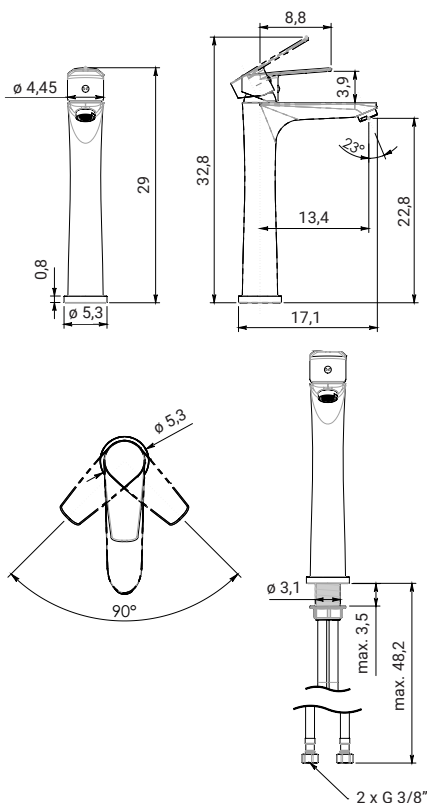
Miscelatore lavabo alto High basin mixer
