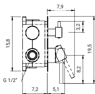
Miscelatore incasso doccia con deviatore Concealed shower mixer with diverter
