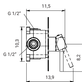
Miscelatore incasso doccia Concealed shower mixer
