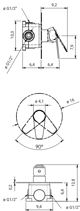
Miscelatore incasso doccia Concealed shower mixer
